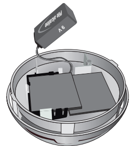
SIRÈNE EXTÉRIEURE AVEC FLASH
